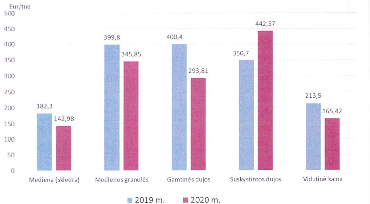
5 pav. Technologinio kuro kainų (Eur/t ne ) palyginimas
