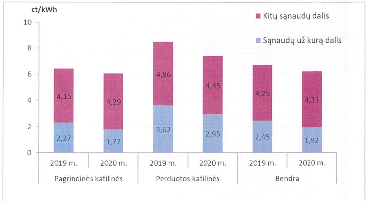
4 pav. Šilumos tiekimo veiklos savikaina, ct/kWh
