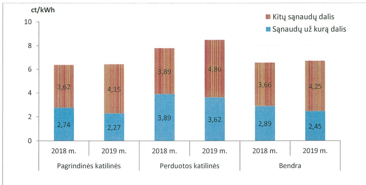
4 pav. Šilumos tiekimo veiklos savikaina
