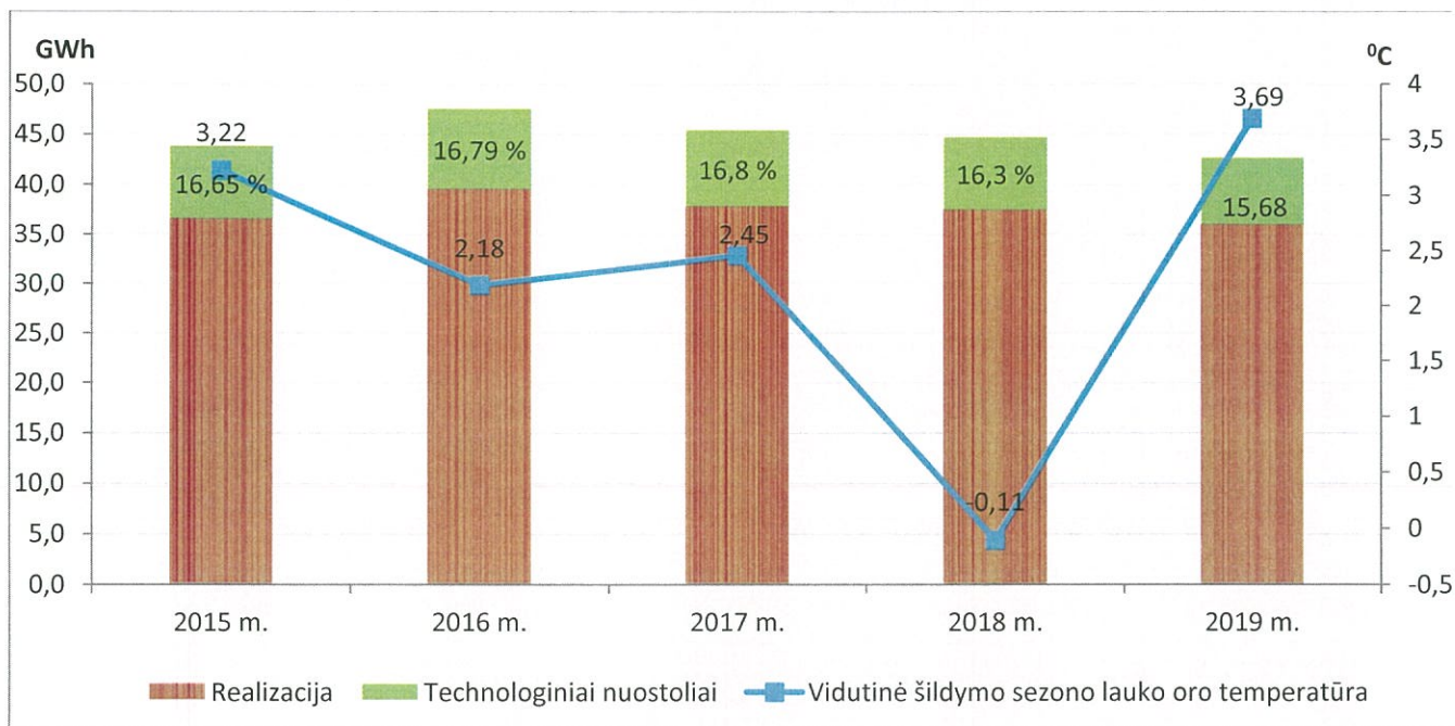
1 pav. Gamybos, realizacijos ir lauko oro temperatūros palyginimas
