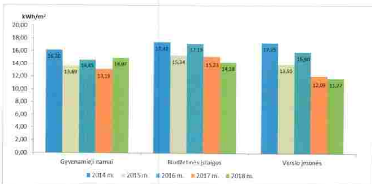
2. pav. Vidutinis šilumos suvartojimas per mėnesį (kWh/m 2 )
