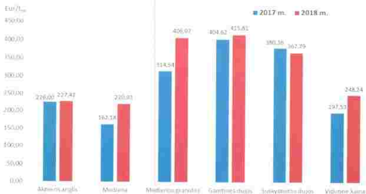
5 pav. Technologinio kuro kainų palyginimas
